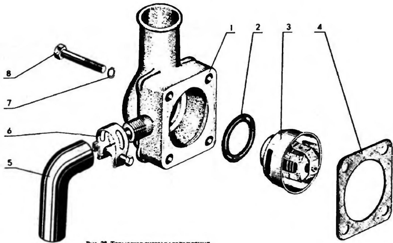
Рис. 28. Термостат системы охлаждения.
