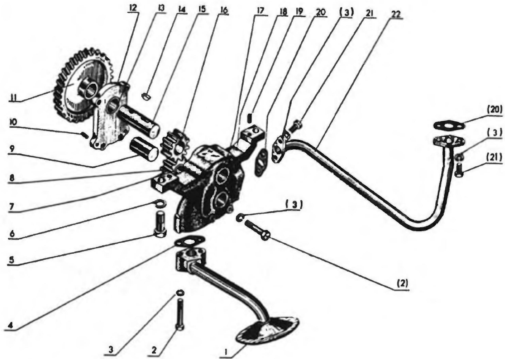
Рис. 32. Приводчик масляного насоса и масляный насос.
