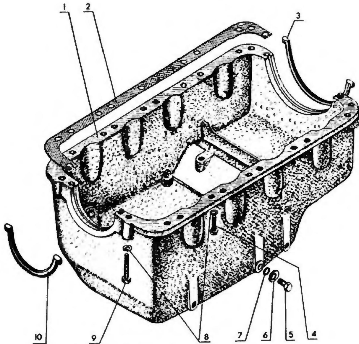
Рис. 31. Масляный картер.
