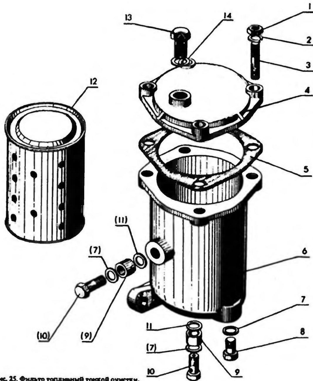
Рис. 25. Фильтр топливный тонкой очистки.
