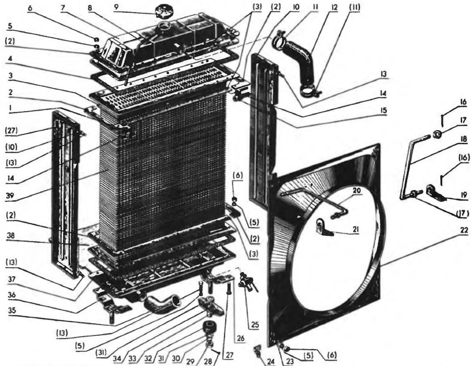
Рис. 27. Водяной радиатор.
